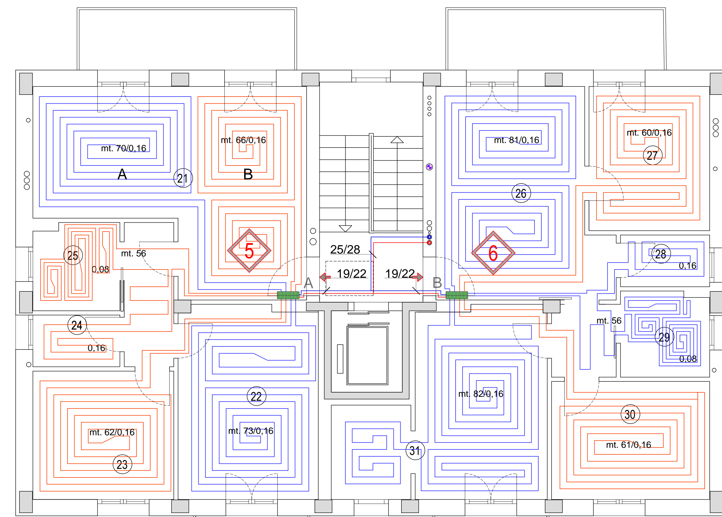
PIANO SECONDO
