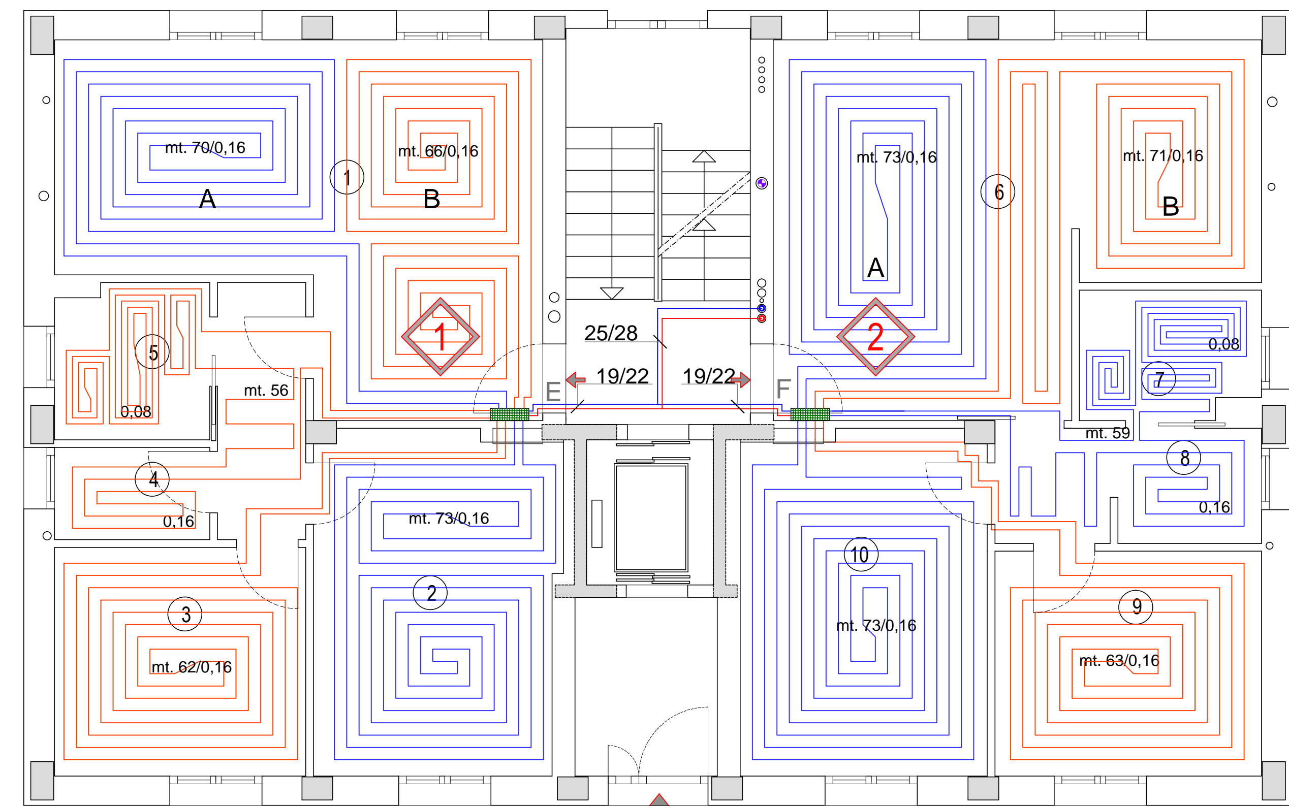
PIANO RIALZATO
