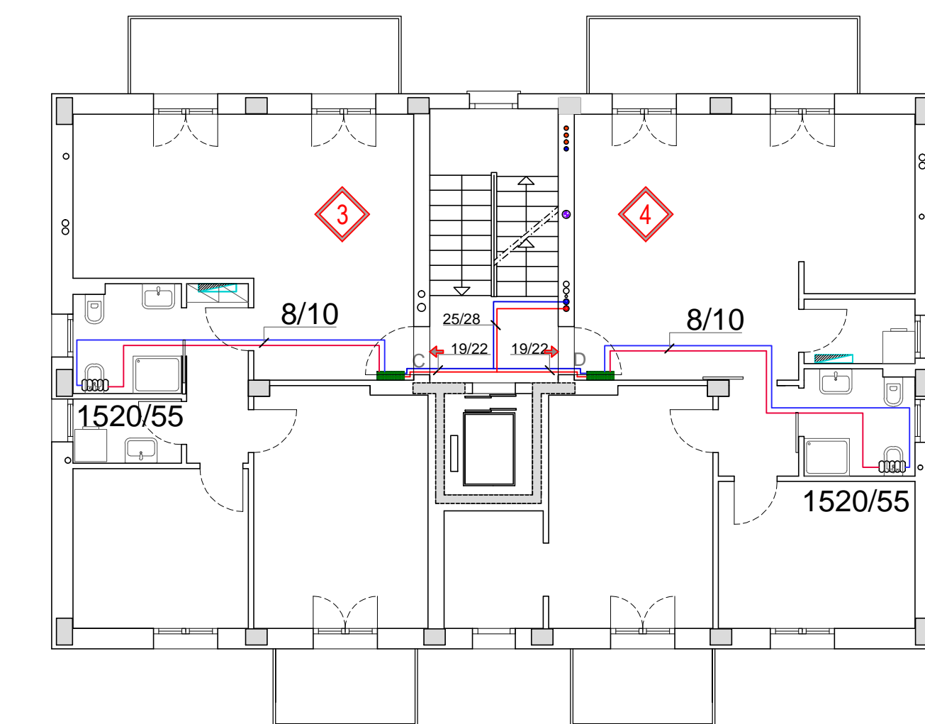
PIANO PRIMO
