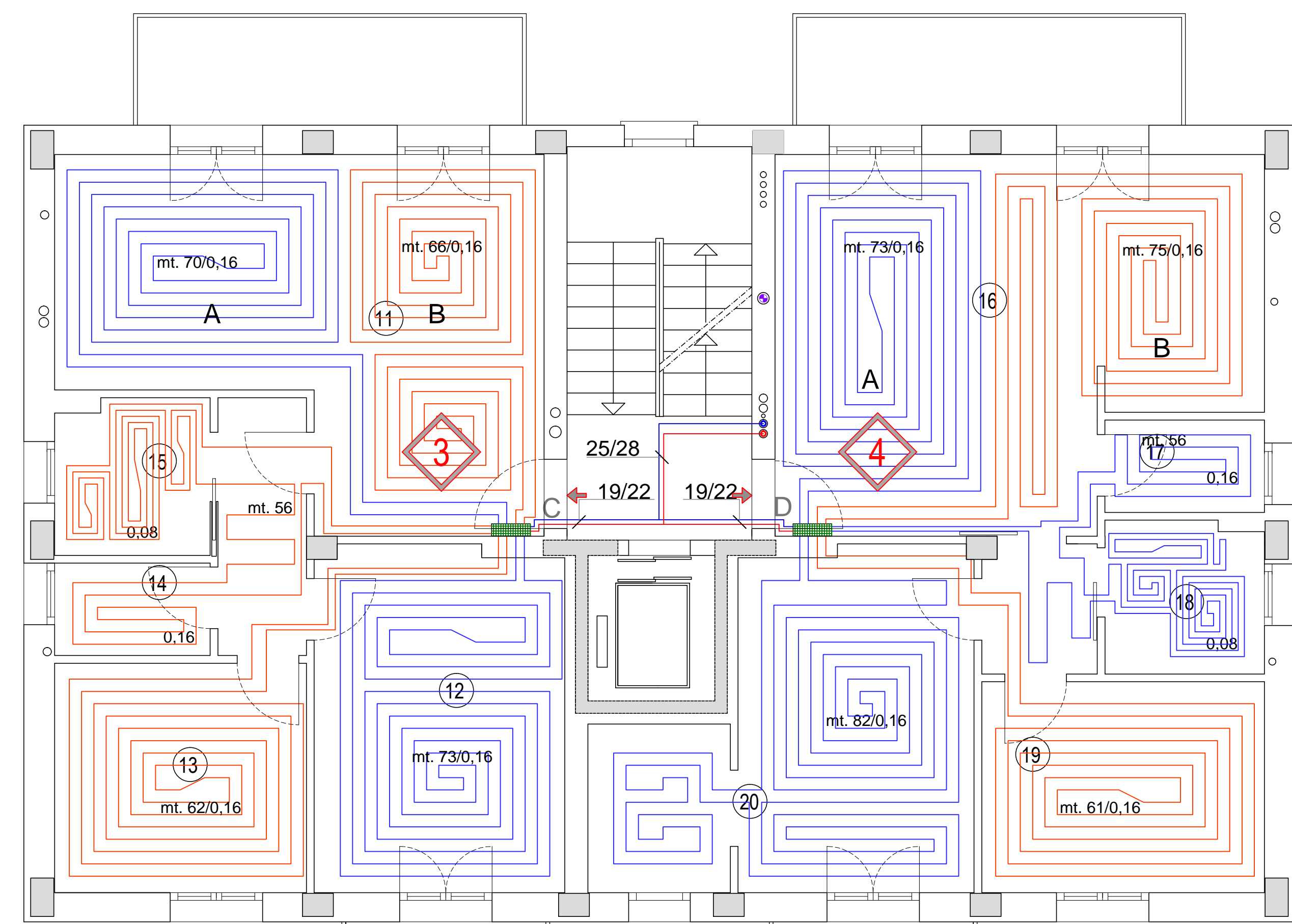
PIANO PRIMO
